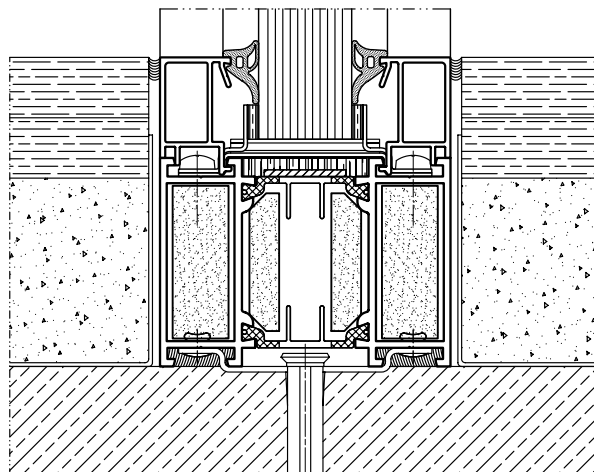
Перегородка без импостов - застройка низ
