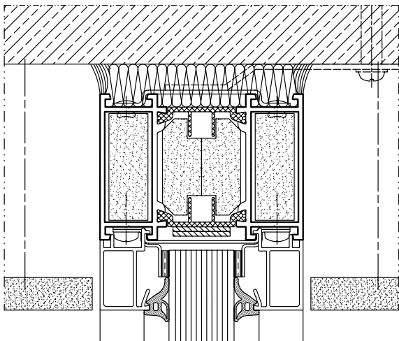
Перегородка без импостов - застройка верх
